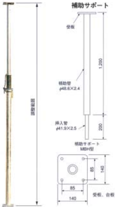
パイプサポートの使用長さの応用と使用強度
