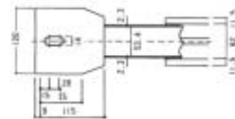
端部詳細図
